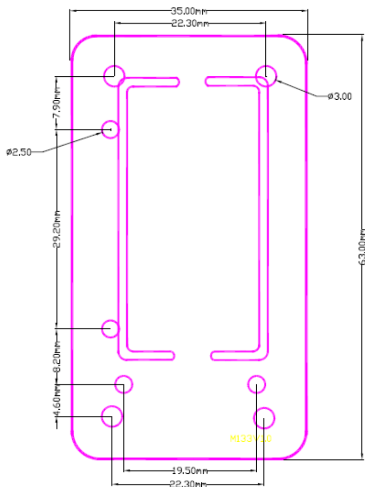
图 1：尺寸图
